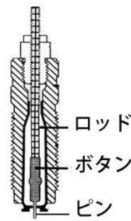
ダイス部品
